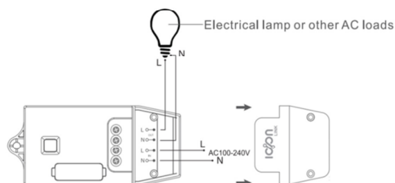
Wiring
