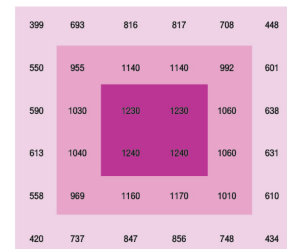
PPFD (area : 120x120 cm, height : 30 cm)
